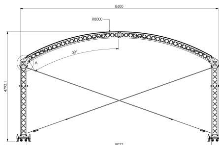
Vue de face – cotes en mm
